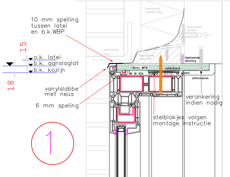
RENOVATIE BOVEN DETAIL VEKA MOTION 82
