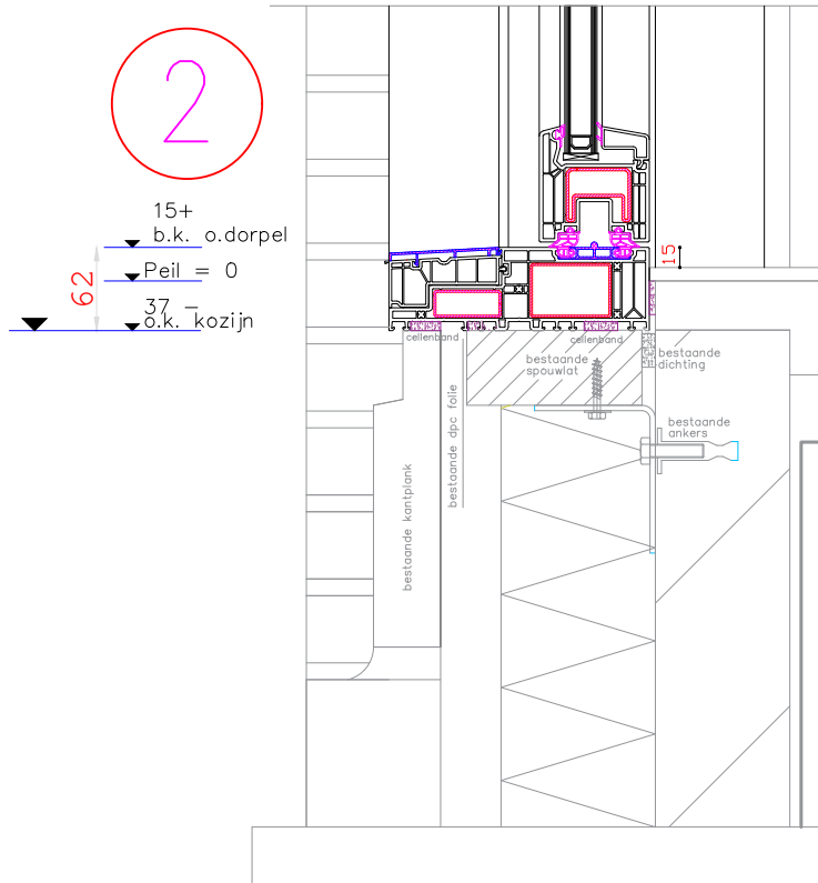
RENOVATIE ONDER DETAIL VEKA MOTION 82
