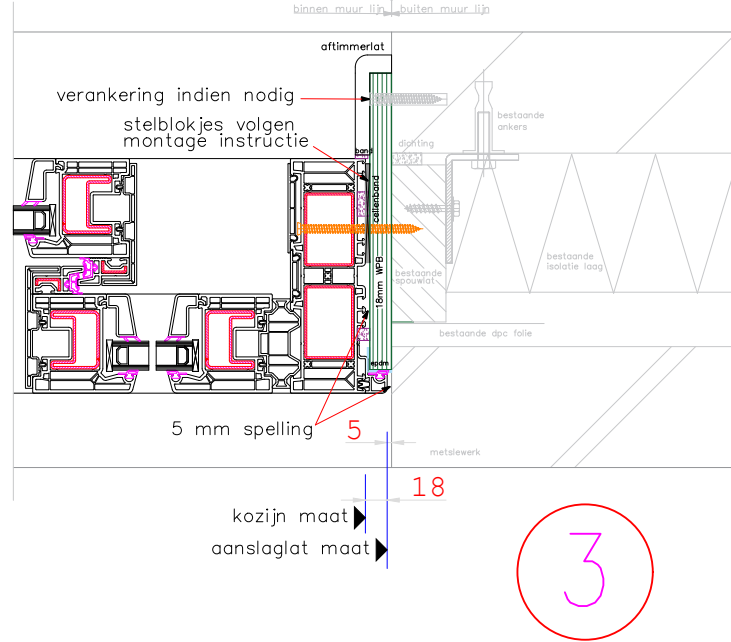
RENOVATIE ZIJ DETAIL VEKA MOTION 82
